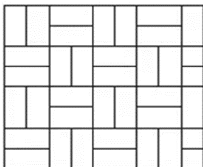
Trama para assentamento e dimensões do paver
